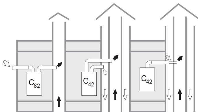
Рис. 6. Примеры систем дымоудаления собранных с помощью отдельных труб. Белой стрелкой обозначен приток воздуха, черной стрелкой поток продуктов сгорания.
