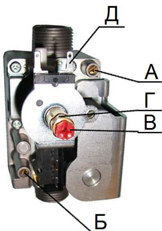
Рис. 9 Регулятор подачи газа
