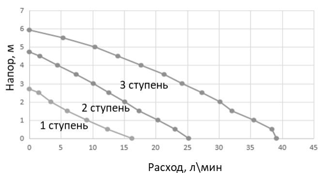
Рис. 13. Напорная характеристика насоса.
