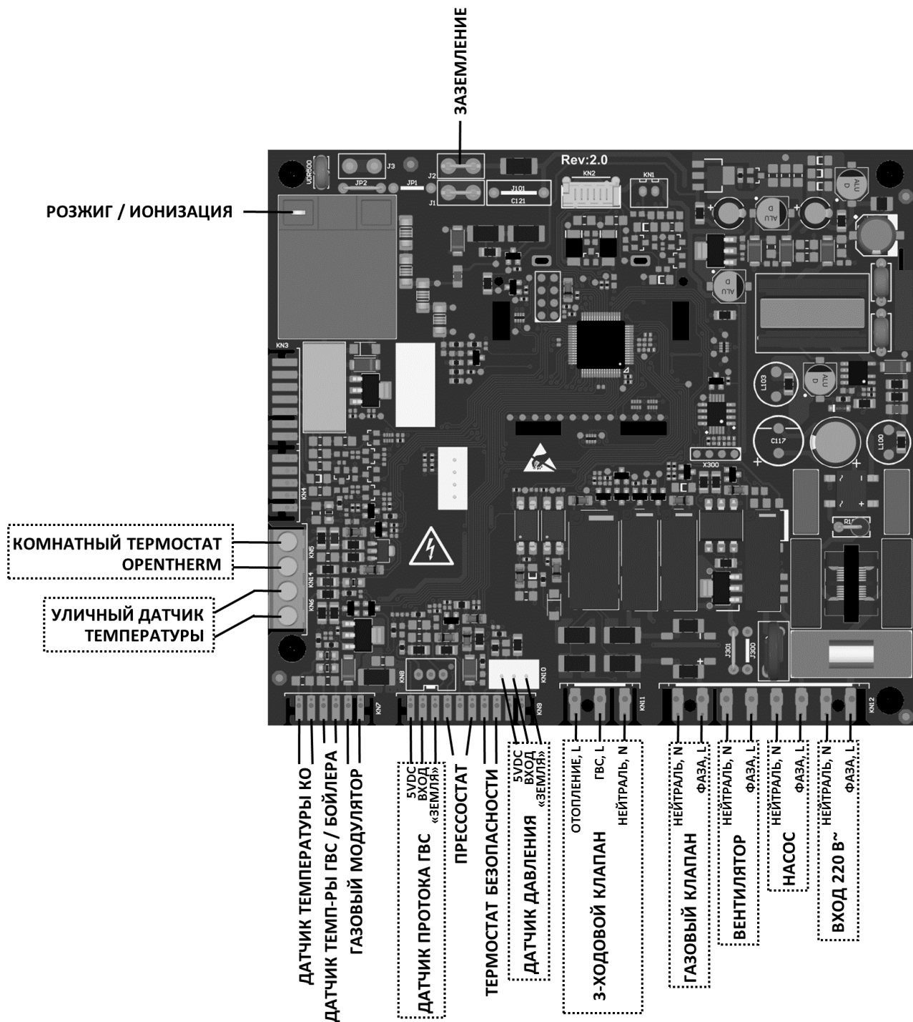
Рис. 14. Электрическая схема
