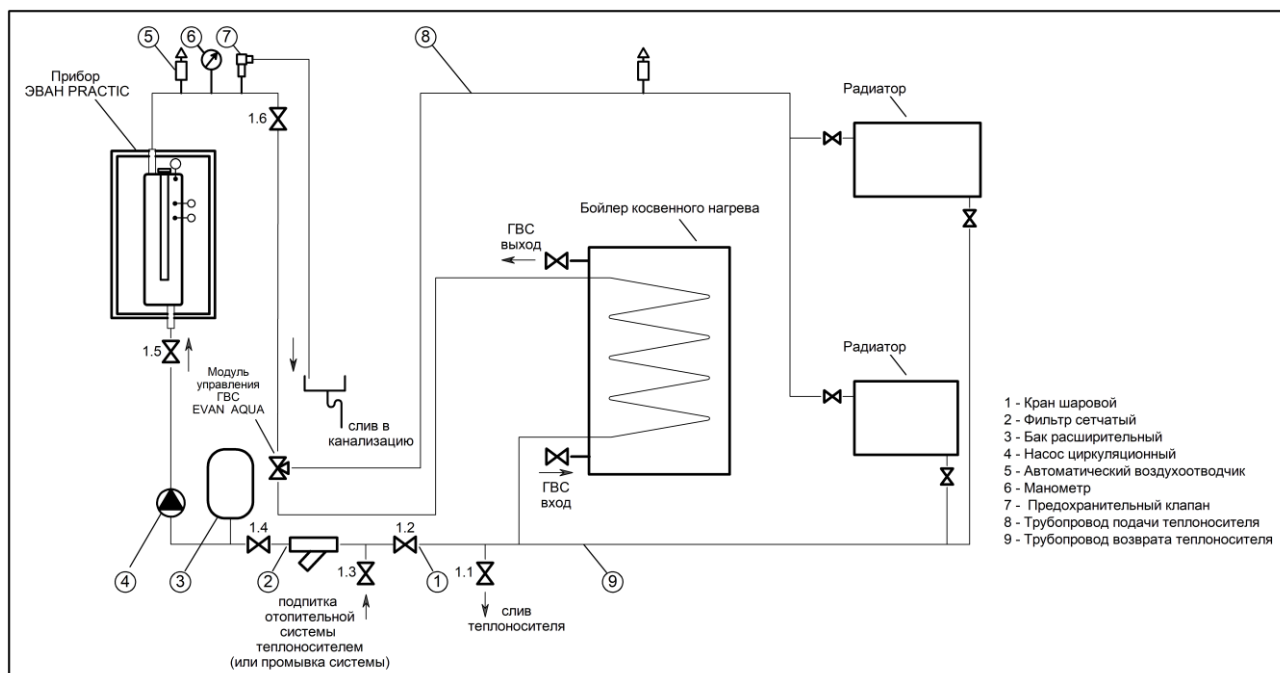
Рисунок 5. Типовая гидравлическая схема системы отопления
