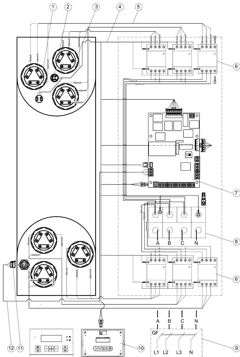
Рисунок 26. Электромонтажная схема подключения EVAN PRACTIC -72...120 к сети 380В
