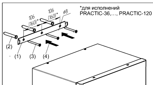
Рисунок 4. Установка котла на вертикальное основание
