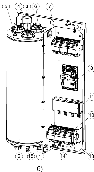
Рисунок 2. Общий вид котла (кожух, блок управления условно не показаны) а) PRACTIC-3...28; б) PRACTIC-36...120
