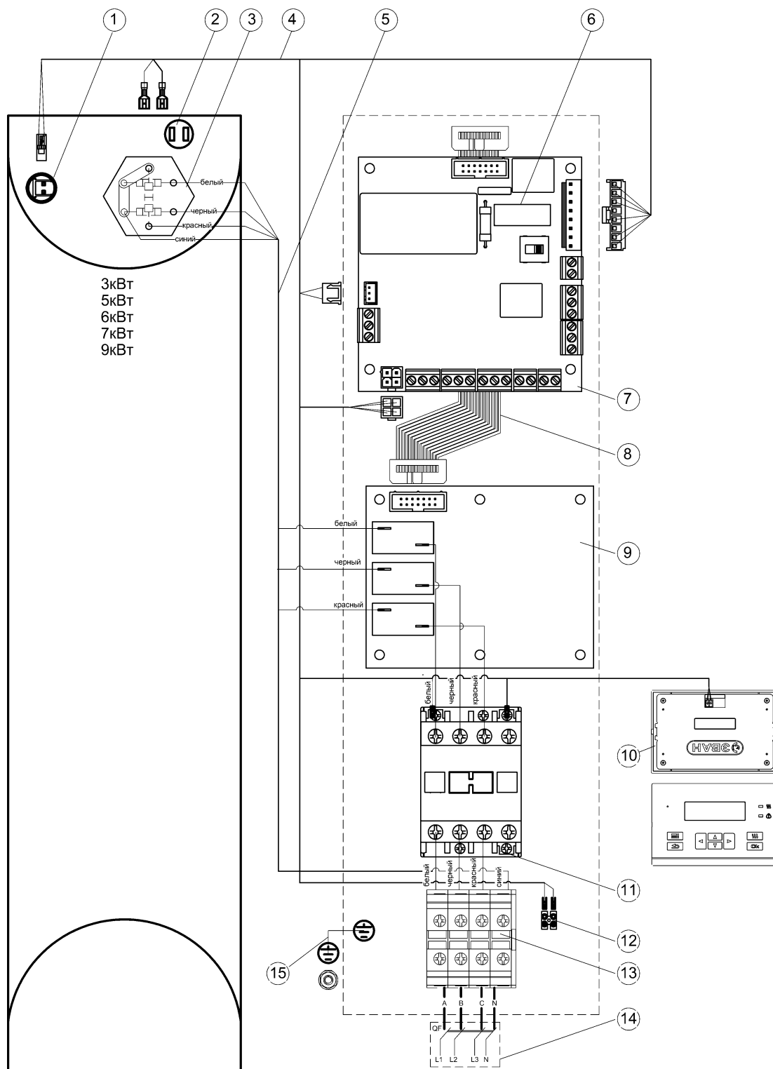
Рисунок 23. Электромонтажная схема подключения EVAN PRACTIC-12; -14 к сети 380В
