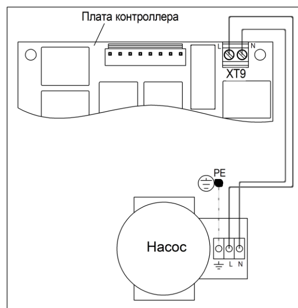
Рисунок 36. Схема подключения насоса к котлу PRACTIC 36-120
