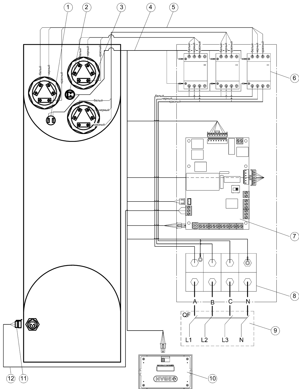
Рисунок 25. Электромонтажная схема подключения EVAN PRACTIC -36; 42; 50; 60 к сети 380В
