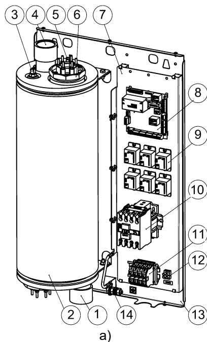
Рисунок 2. Общий вид котла (кожух, блок управления условно не показаны) а) PRACTIC-3...28; б) PRACTIC-36...120
