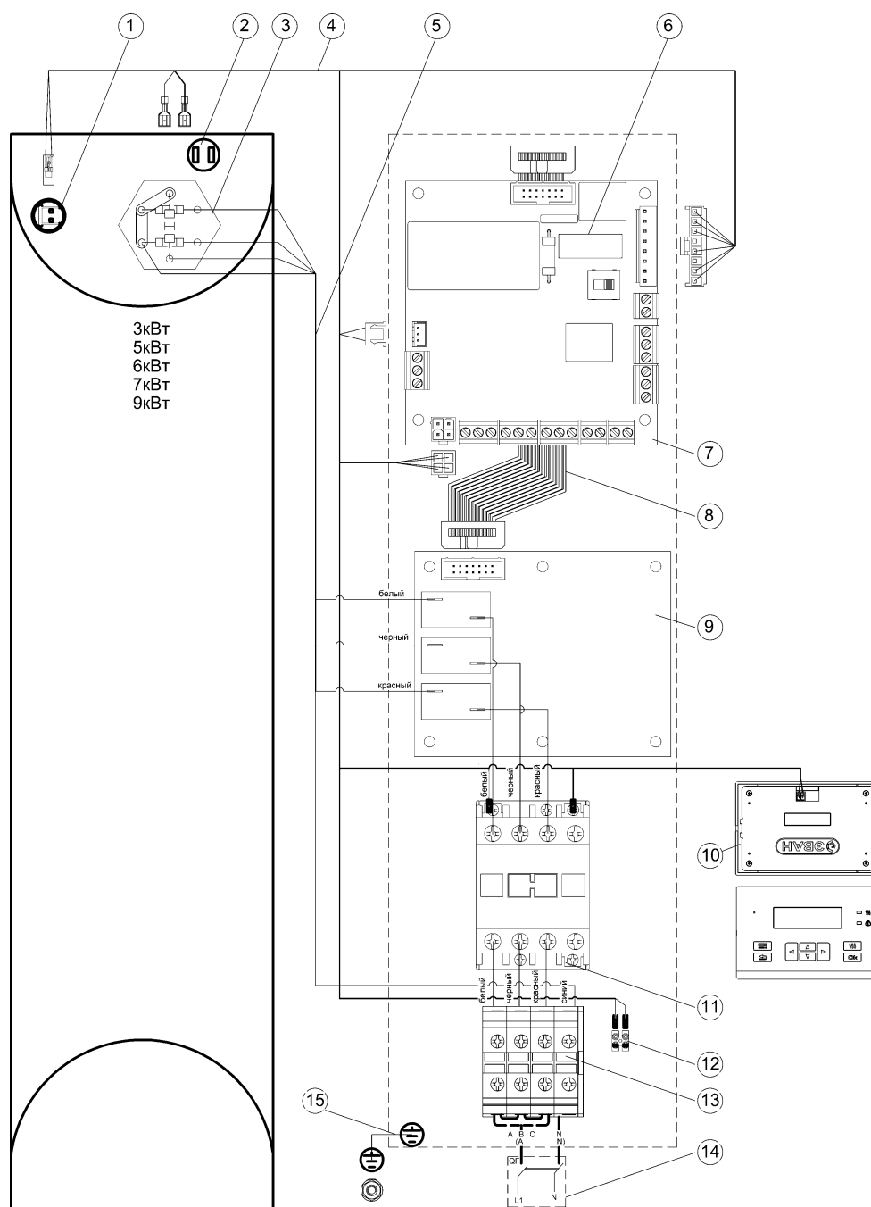
Рисунок 21. Электромонтажная схема EVAN PRACTIC-3...9 к сети 220В
