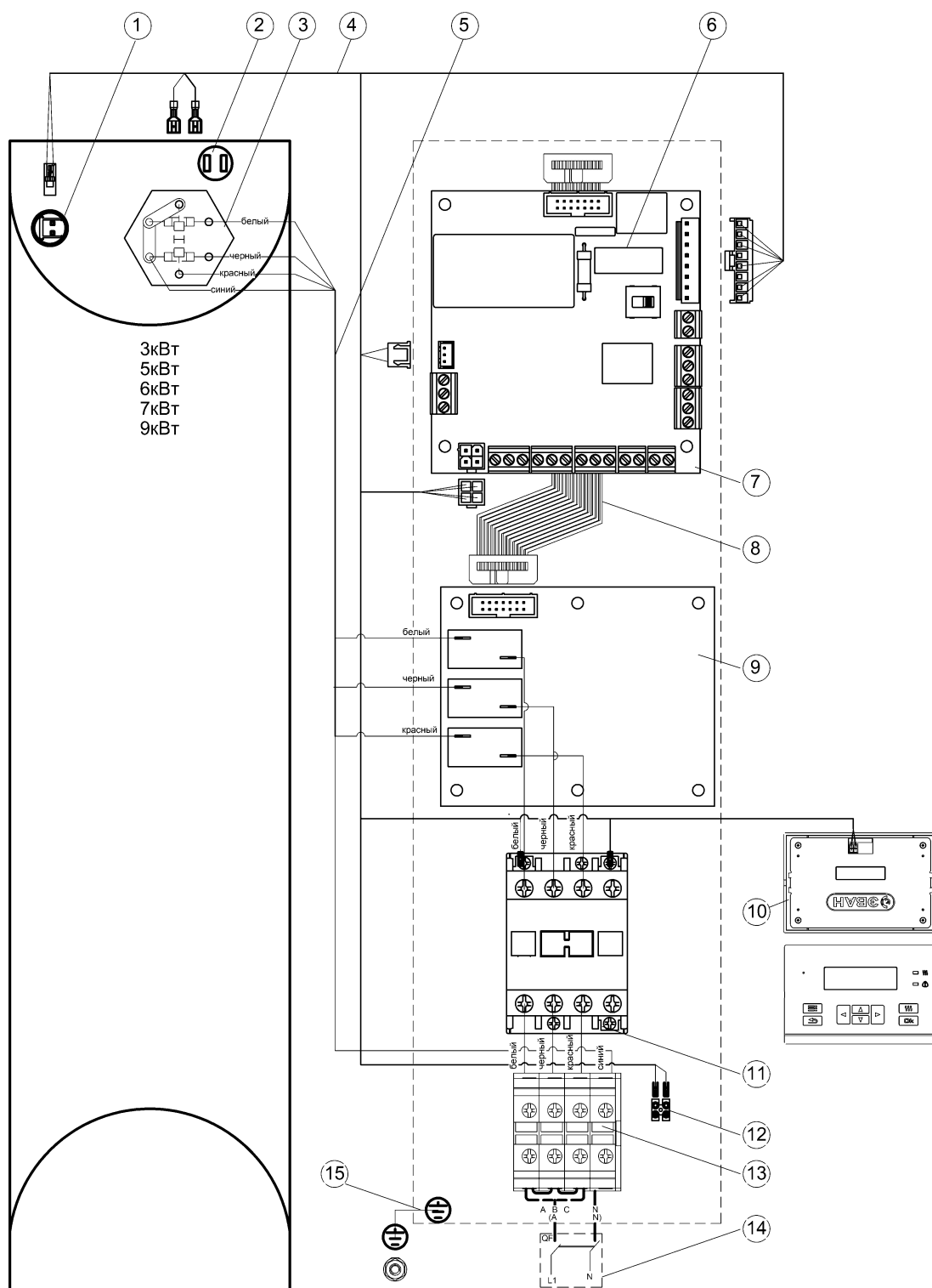
Рисунок 22. Электромонтажная схема подключения EVAN PRACTIC -3...9 к сети 380В
