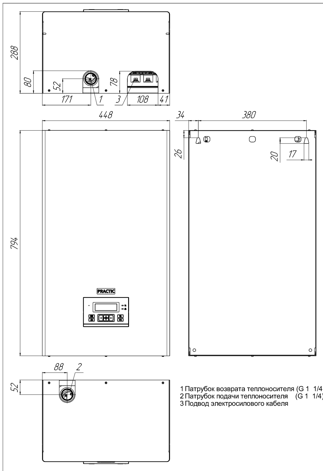
Рисунок 20. Габаритные и присоединительные размеры котлов EVAN PRACTIC-36,....., PRACTIC-120
