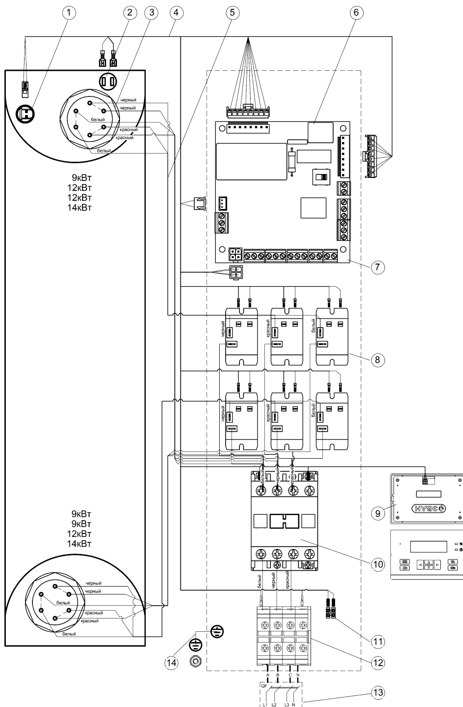
Рисунок 24. Электромонтажная схема подключения EVAN PRACTIC -18...28 к сети 380В
