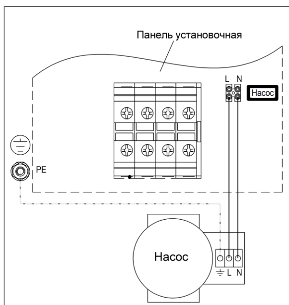
Рисунок 34. Схема подключения насоса к котлу PRACTIC 3-28
