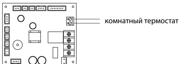
основная плата управления
