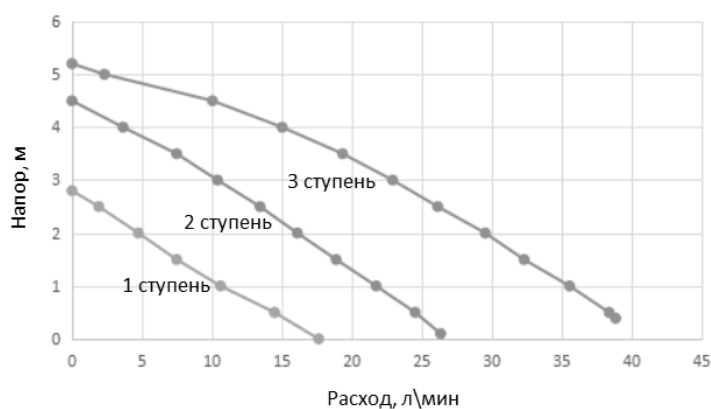
Рис. 13. Напорная характеристика насоса.
