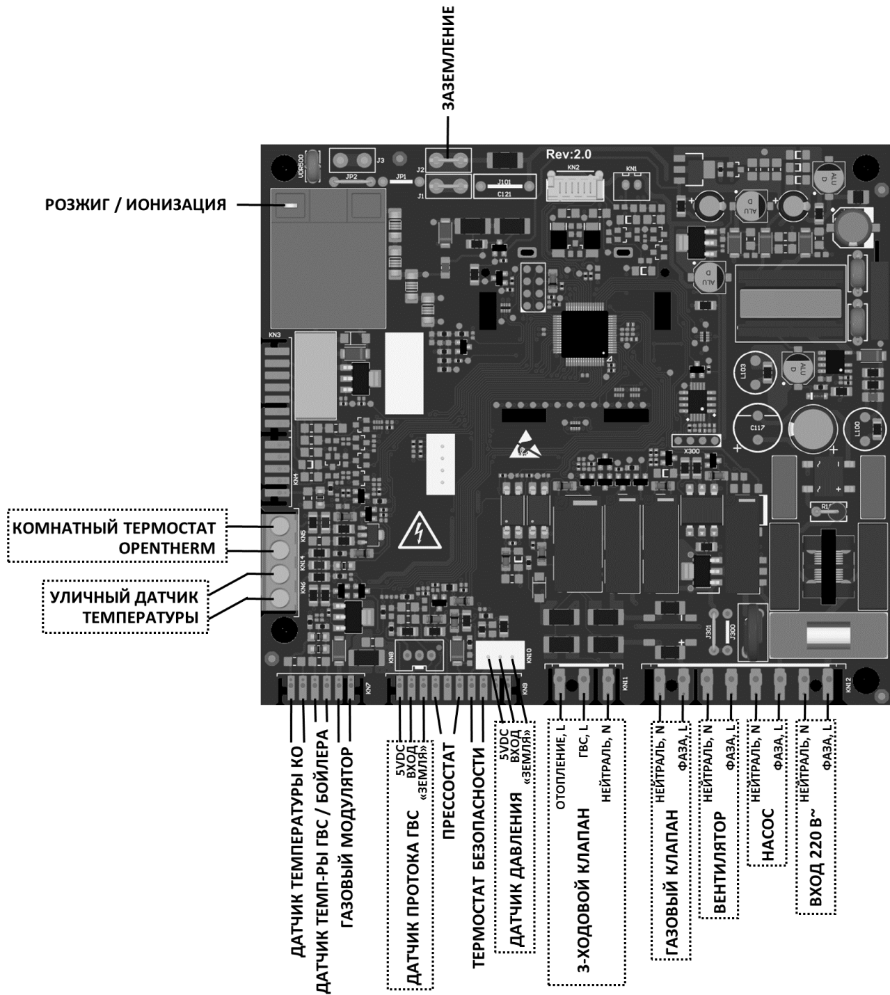
Рис. 14. Электрическая схема
