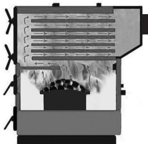
Рис. 5. Схема движения дымовых газов в трехходовом теплообменнике для котла VLK PRK 160-1500.
